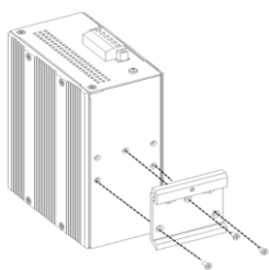
Figure 7. DIN Rail
